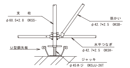
脚部詳細図 (1:20)
