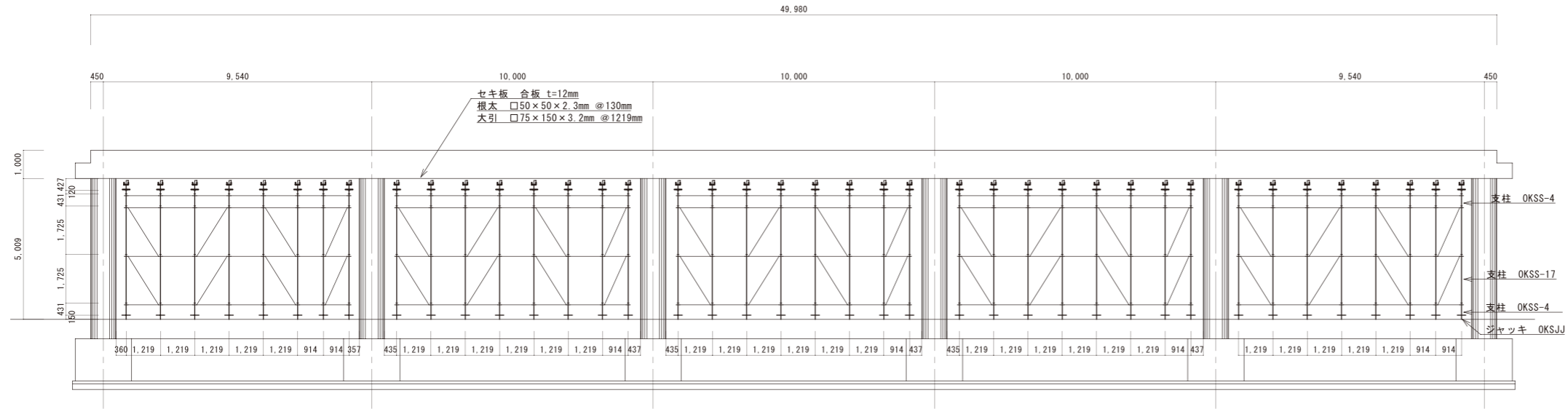
A-A S=1:100
