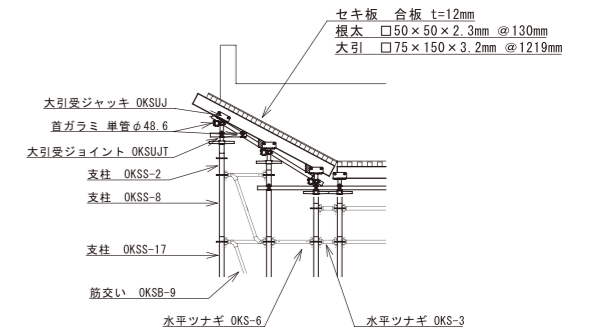
支保工上部詳細 S=1:50
