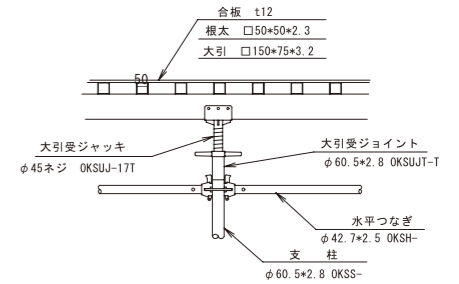
頭部詳細図 (1:20)
