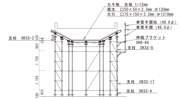
C-C S=1:100
