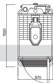
平面図
