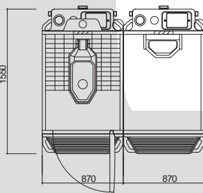
平面図
